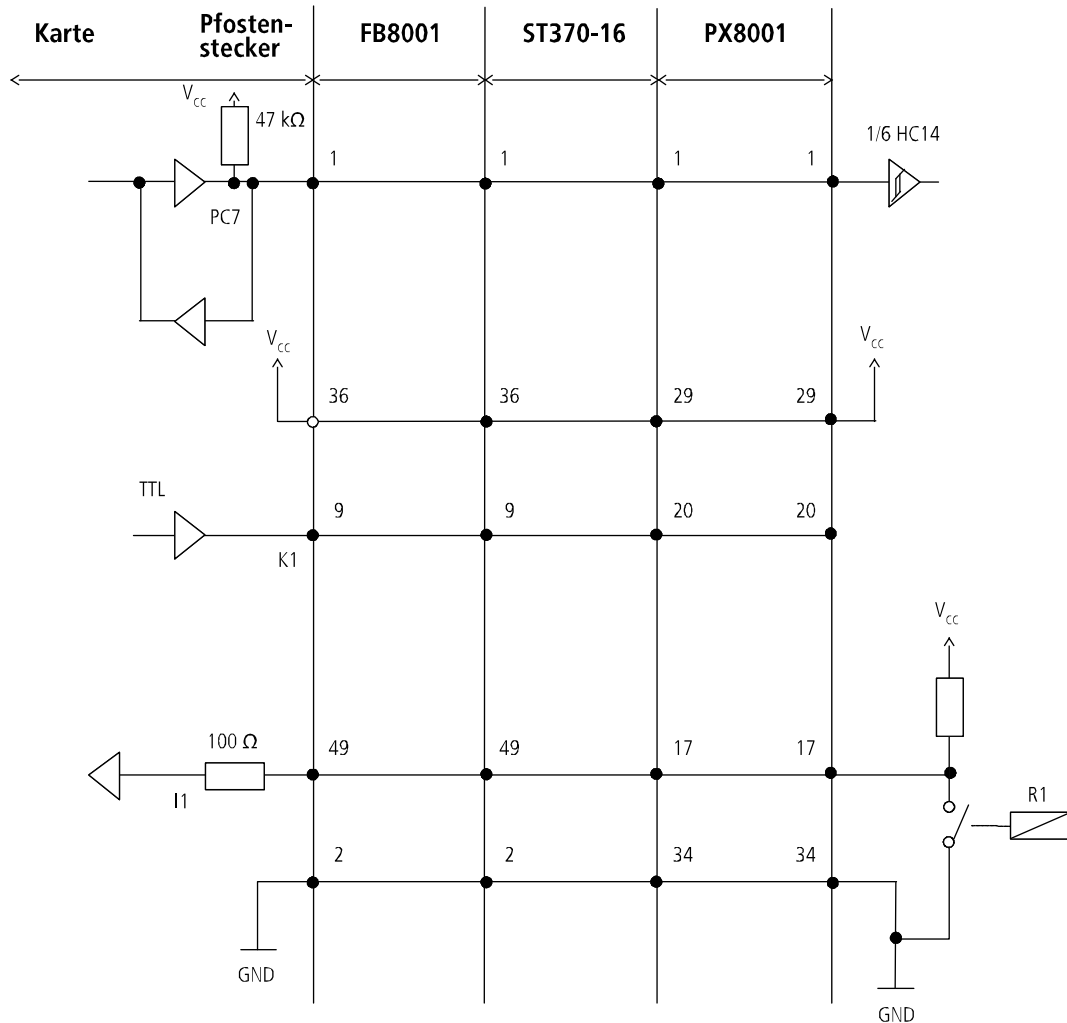
Abb. 1-6: Anschlussbeispiel
