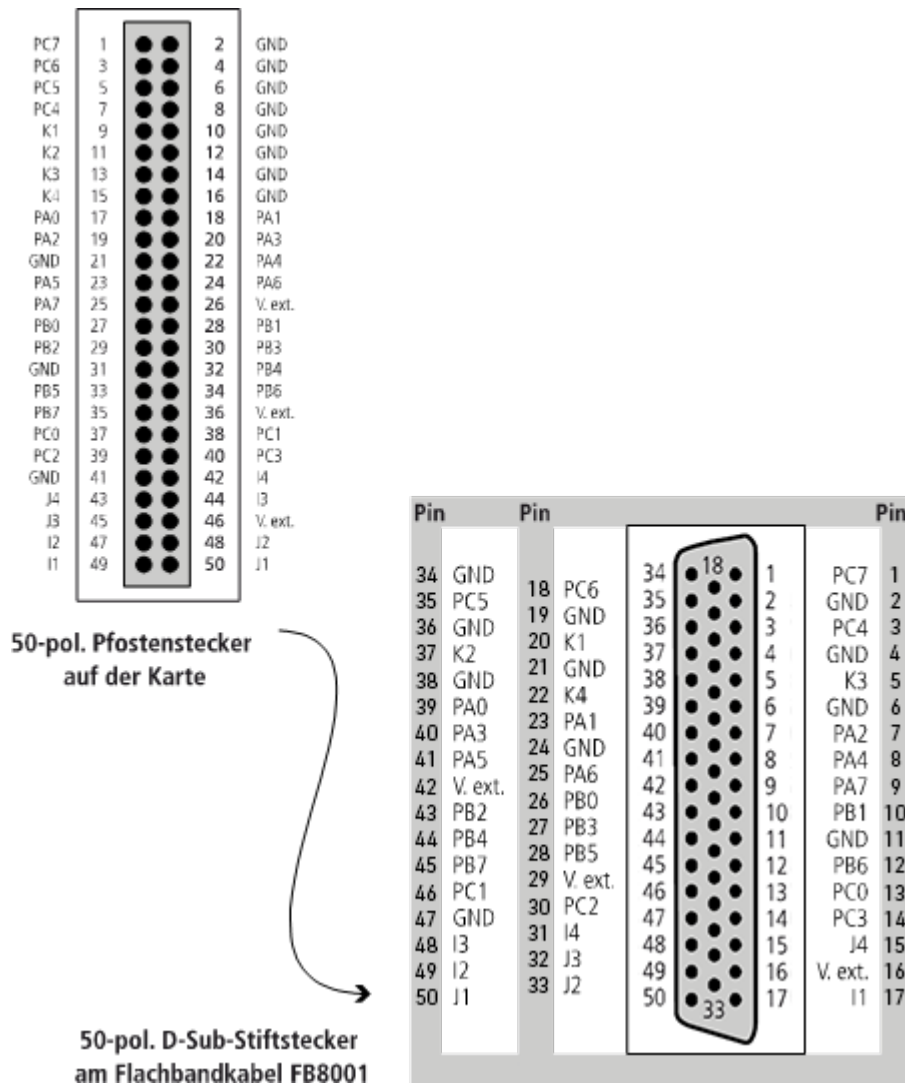
Abb. 1-2: Steckerbelegung: 50-pol. Pfostenstecker und 50-pol. D-Sub-Stiftstecker
